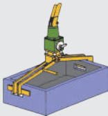
トレークランプ治具
